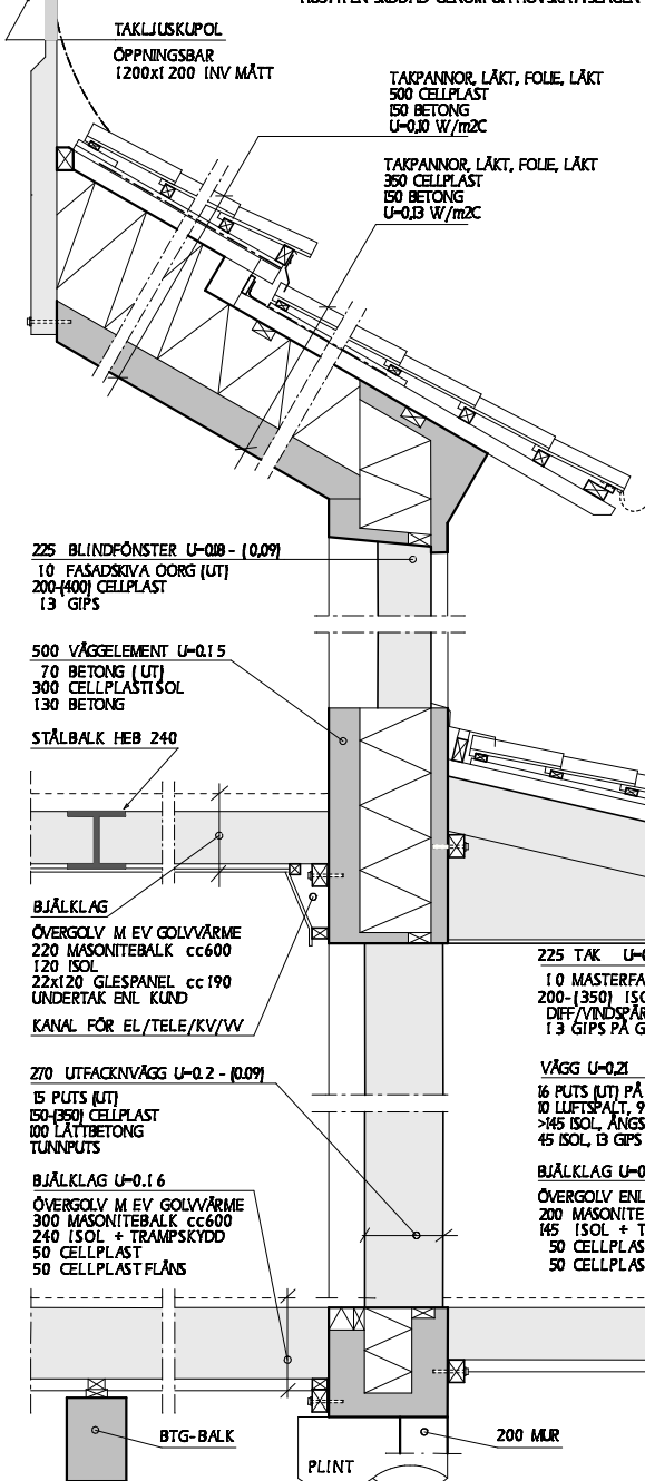
SEKTION HUSTYP V1 *HUSTYP V2
