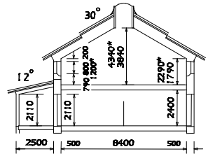
SEKTION HUSTYP V1 *HUSTYP V2
